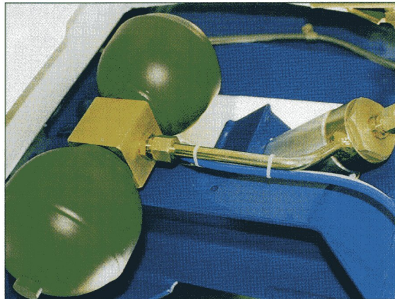
MONTAGE À DOUBLE SPHÈRES
