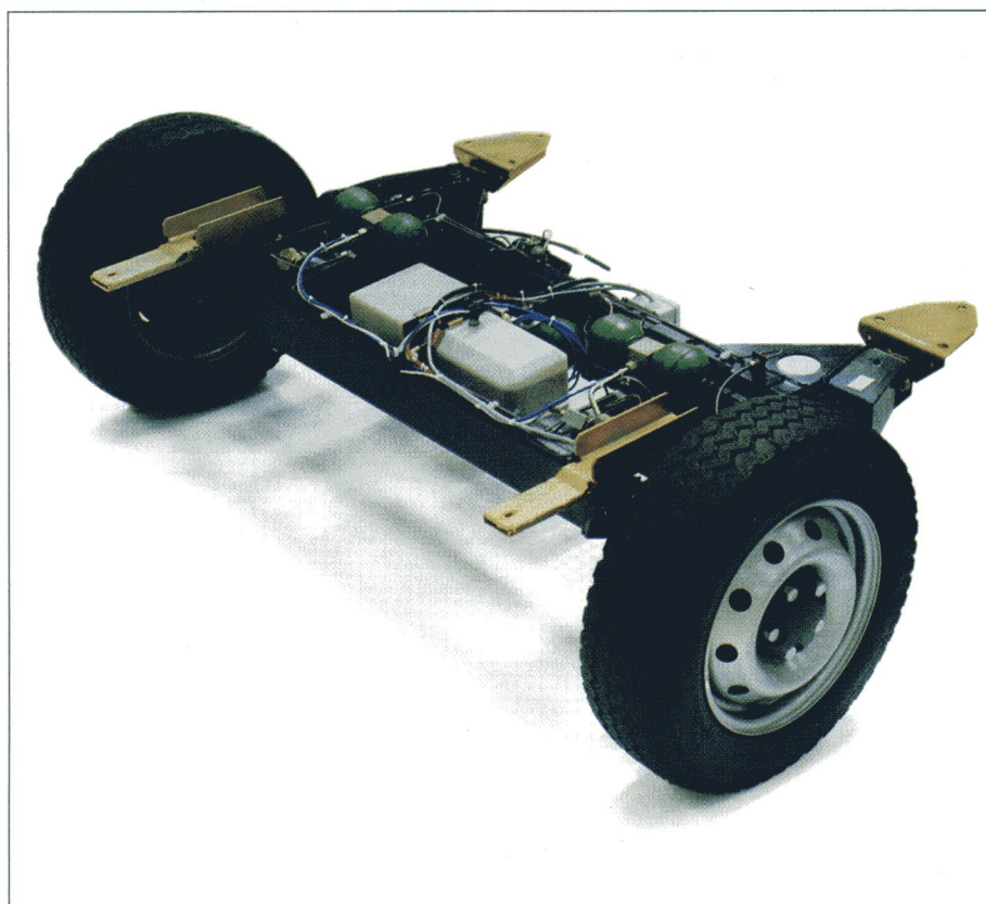
UNITÉ ARRIÈRE DE SUSPENSION HYDROPNEUMATIQUE
